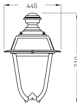
Disegno quotato (mm)
